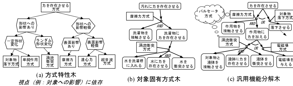
図 3 機能達成方式の is-a 階層以外の構造化の例
