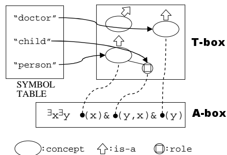
図 1 KRYPTON における T-box と A-box [Brachman 83]
